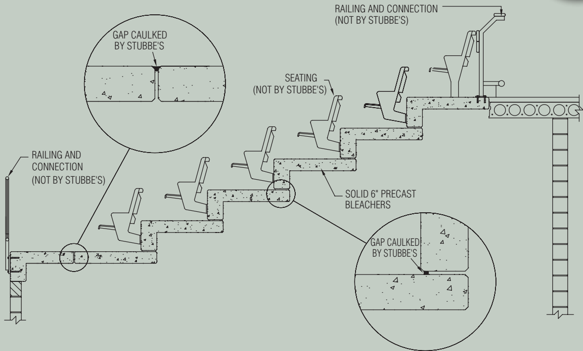
Bleacher Section A-A
